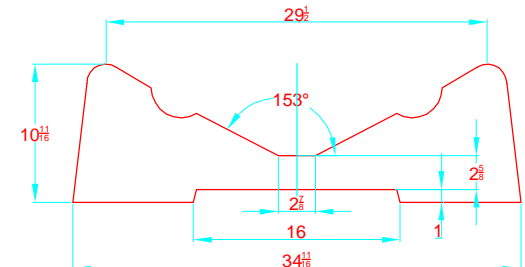
TRANSVERSAL SECTION "B" SECCION TRANSVERSAL "B"
